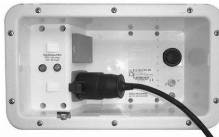
Sähkökotelo ulkopuolelta
