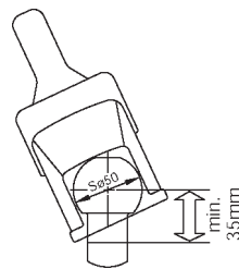
Kuglehals, trækkøretøj
