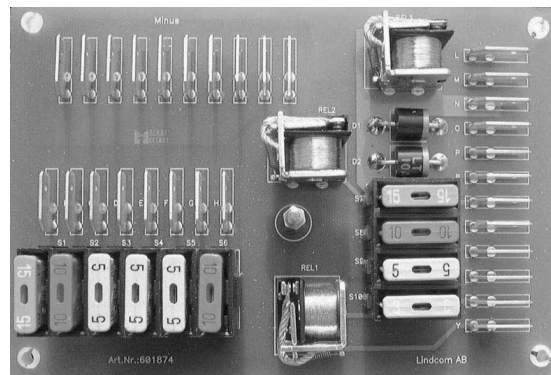
Kredsløbskort med sikringer
