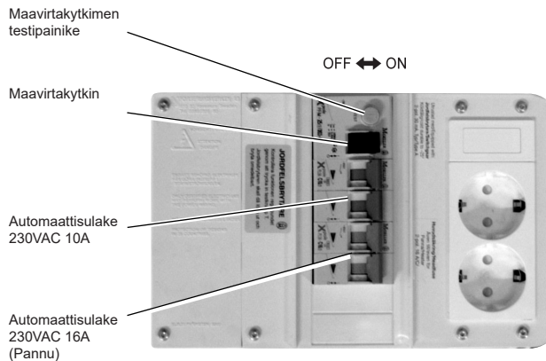
Sähkökotelon takaosa
