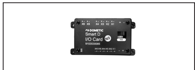
Väyläjärjestelmän yksiköt N1-N6 on nimetty: Dometic Smart D I/O Card.
