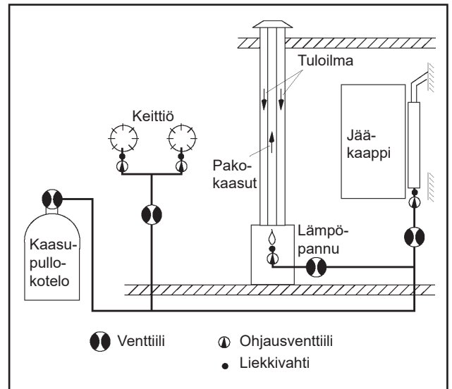
Kaaviokuva nestekaasujärjestelmästä.
