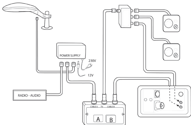
Schematisch overzicht van het antennesysteem.
