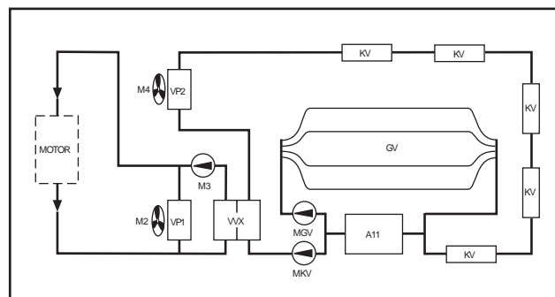
Halvintegret bil med AGS II Pro (med shuntventil).
