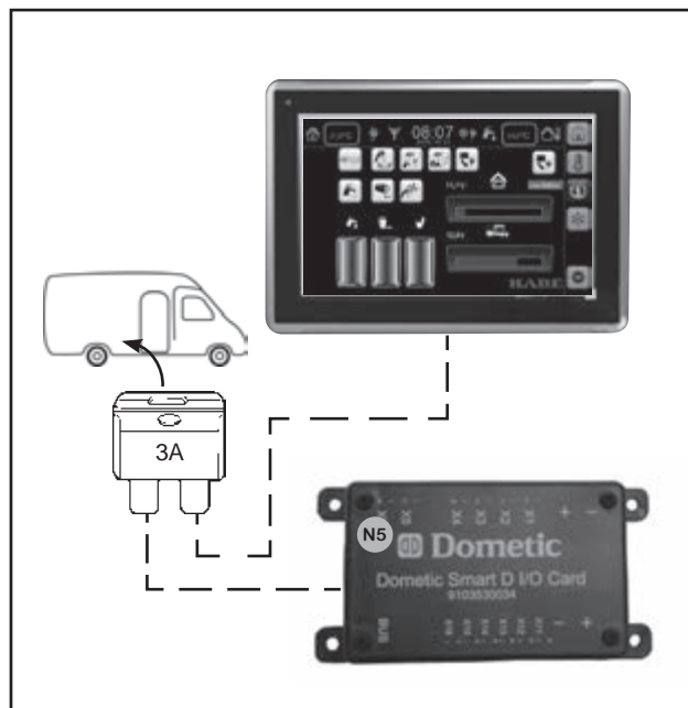
Sikringen til betjeningspanelet er plassert ved enheten ved siden av døren.
