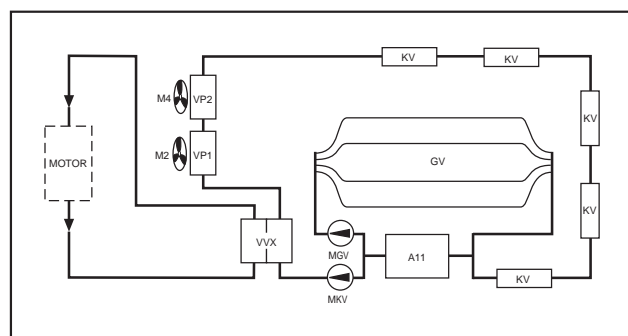
Helintegret bil med AGS II Pro (med shuntventil).
