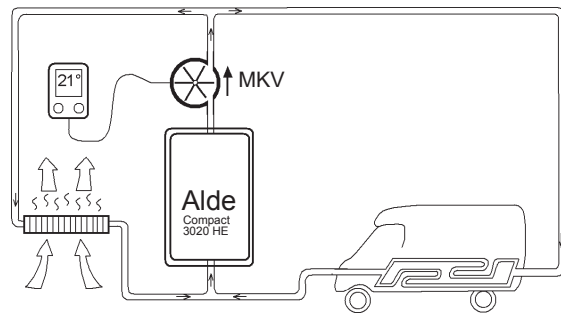
Abb. 1: Schematische Darstellung des Heizsystems im Wohnteil.
