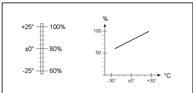
Batteriekapazität bei unterschiedlichen Temperaturen.
