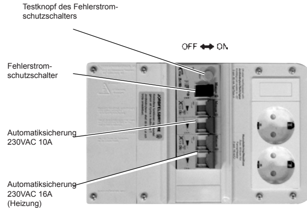
Rückseite des Schaltkastens
