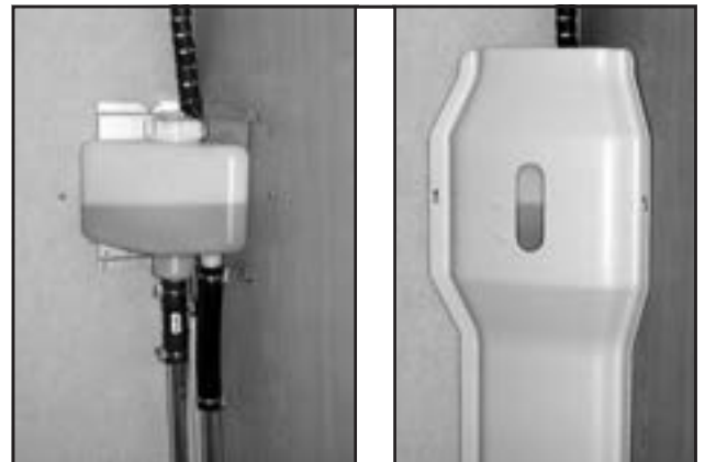
Expansionskärlet och täckskivan med inspektionshål.
