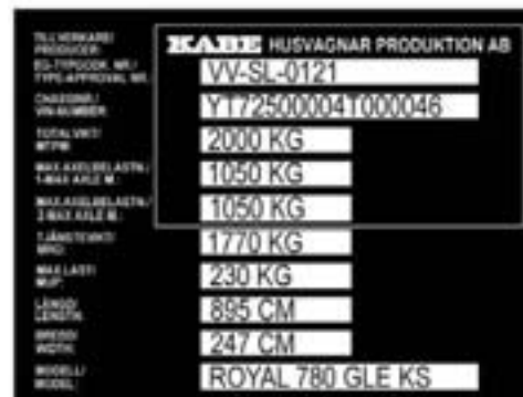
Yhdistetty tyypikilpi ja katsastuskilpi Ruotsin markkinoita varten.
