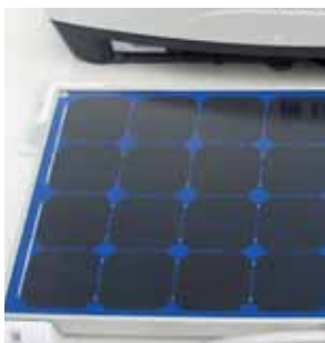
Solarzellenpanel Y0163 85 W einschl Regler und Überwachungspanel
