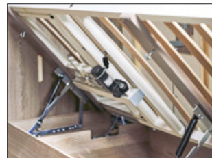
Bett mit elektrisch verstellbarem Kopfteil (Serienmäßig im Imperial, nicht für E9-Bett)
