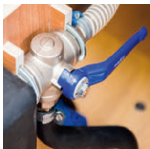
PARALLELKOPPELING GRIJSWATERTANK
