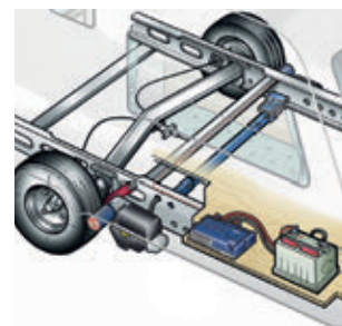
TRUMA MOVE CONTROL TANDEMASSER (X0216) EENASSER (X0217) 4 MOTOREN (X0282)
