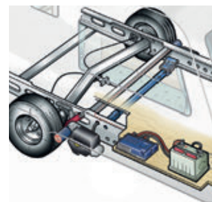
TRUMA MOVE CONTROL BOOGIE (X0216) ENKEL (X0217) 4 MOTORER (X0282)
