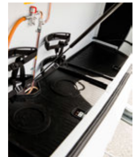
Formgegossene Schutzmatte im Gaskasten
