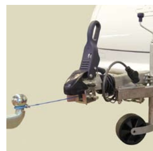
Puller Winch (X0204) För säker uppkoppling. Puller Winch passar de flesta kulkopplingar och manövreras med hjälp av ett spårskafat med 17 mm hylsa.
