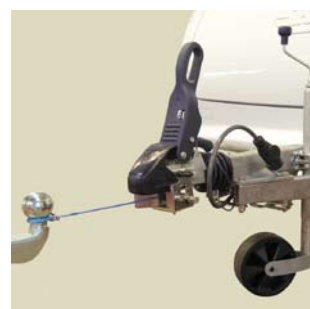
Puller Winch (X0204) Für das sichere Ankoppeln. Puller Winch ist für die meisten Kugelkupplungen geeignet und wird mit Hilfe eines Sperrschiffs mit 17-mm-Hülse bedient.
